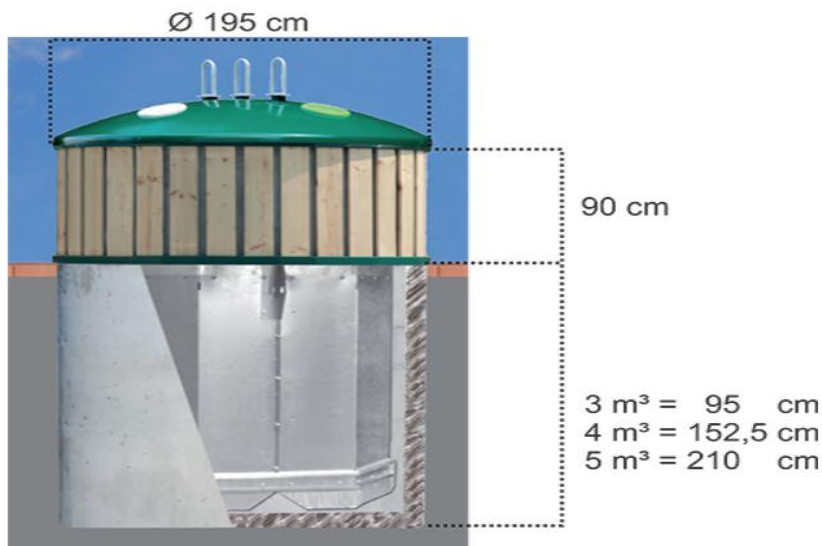
Figura 01 – Especificações do Container Semienterrado
