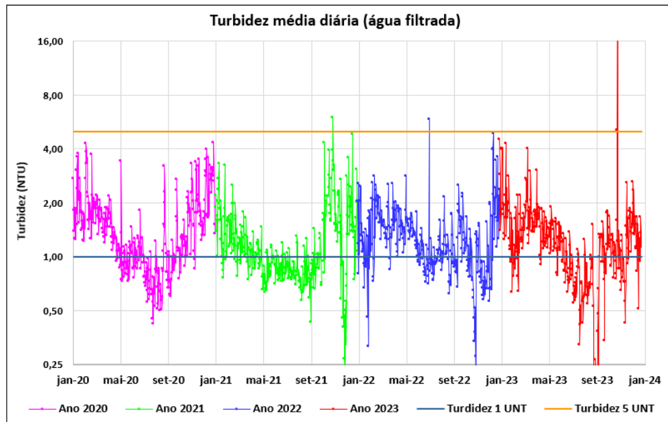
Figura 10: Turbidez Média Diária - Água Filtrada
