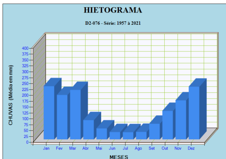
Figura 2: Hietograma Guaratinguetá
