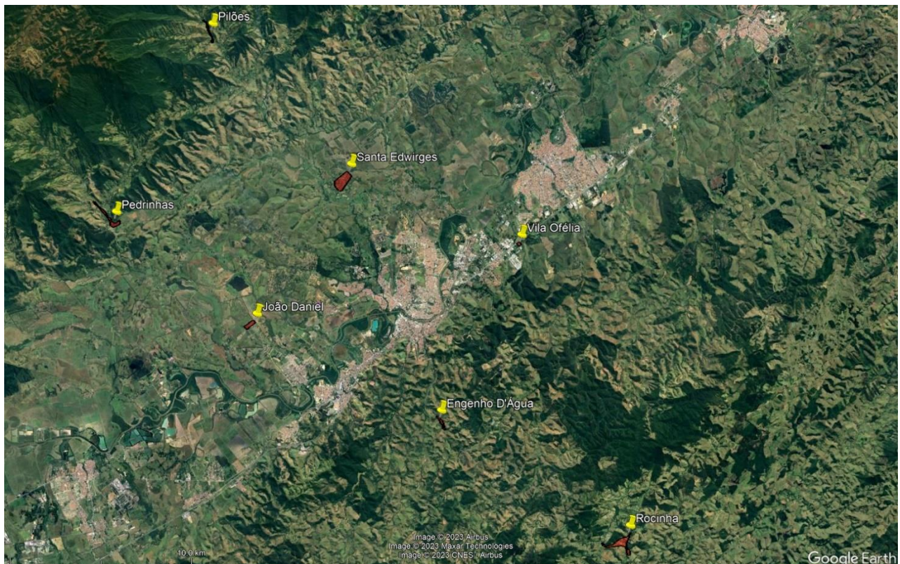
Figura 17: SAA Isolados
